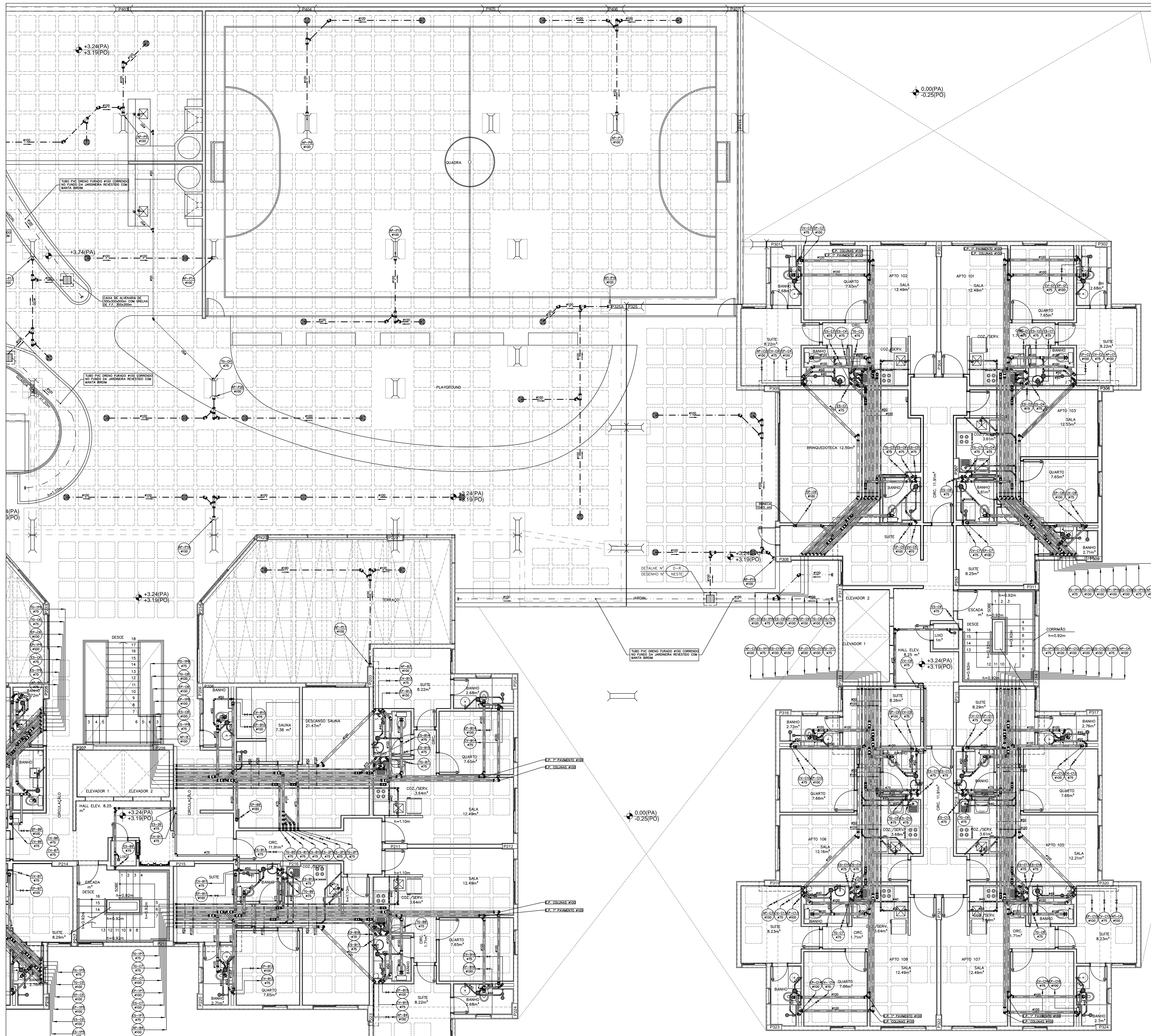
PLANTA BAIXA - 1º PAVIMENTO TRECHO 2
